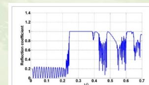
Спектр отражения рассматриваемого фотонного кристалла (ТЕ поляризация).
