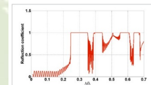
Спектр отражения рассматриваемого фотонного кристалла (ТМ поляризация).
